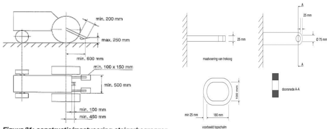
Figuur 31: constructie/maatvoering steigerbegrenzer
